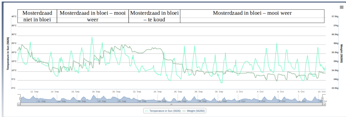
Figuur 2: Temperatuur en gewichtsveranderingen tijdens maand september 2018
